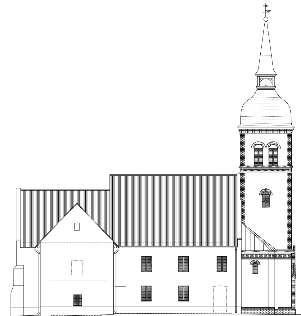
ELEWACJA PÓLNOCA
